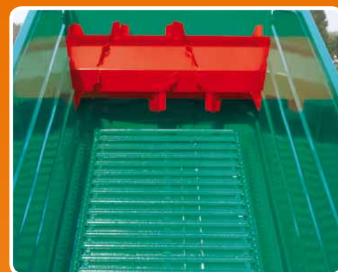
Rullo maggiorato dosatore e frantumatore Increased beater dispenser and crusher
